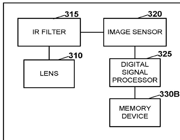
CAMERA MODULE 305
